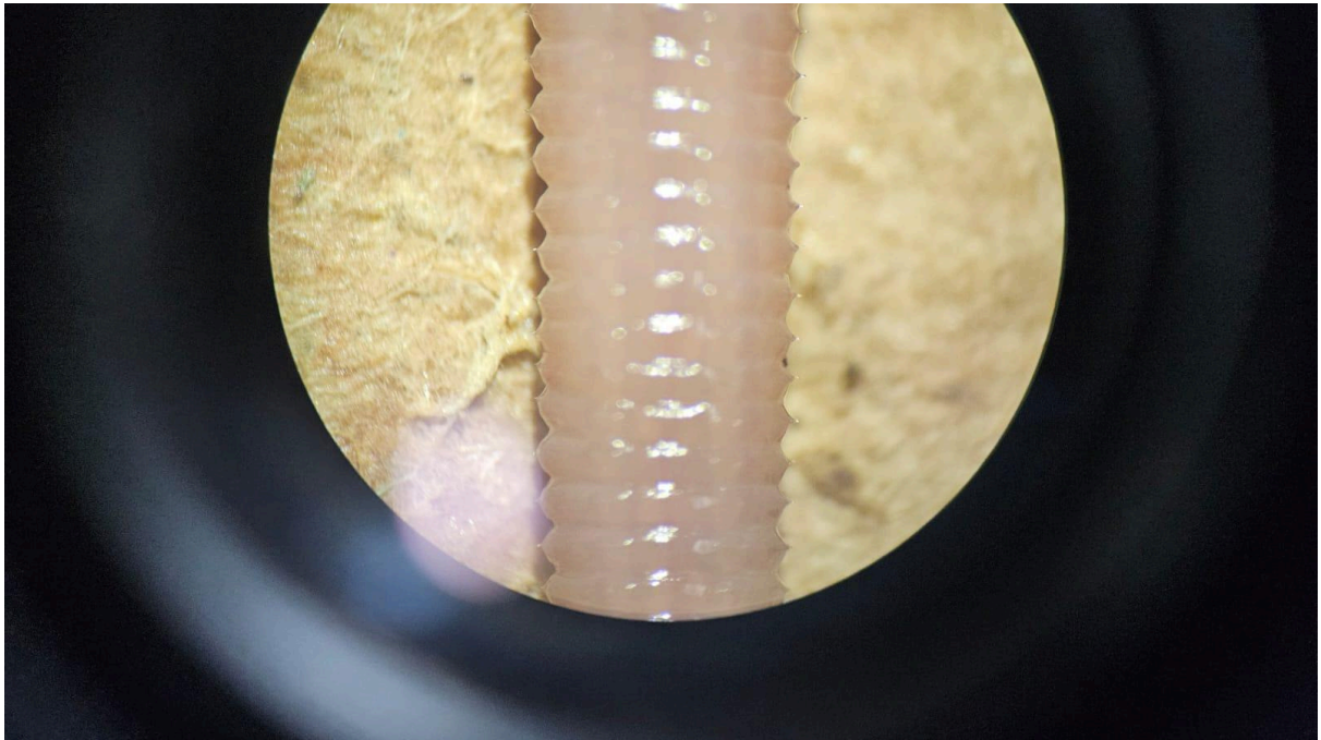
Figura 1: Quetas da Oligochaeta
