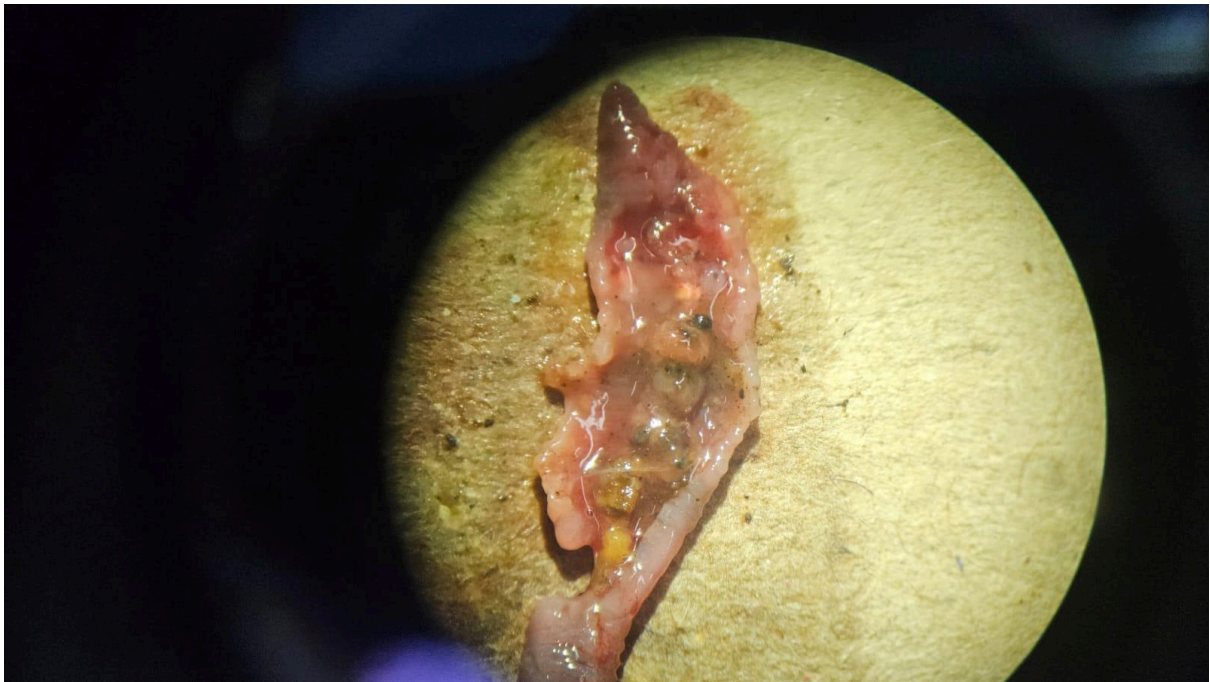
Figura 2: estruturas internas da Oligochaeta
